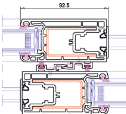
Sección central puerta
